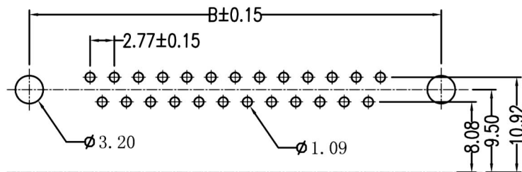
P.C.B. PLYOUT
