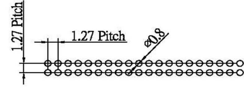
P.C.Board Layout
