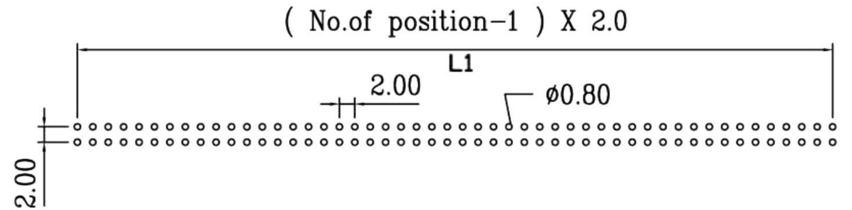
P.C.B.layout
