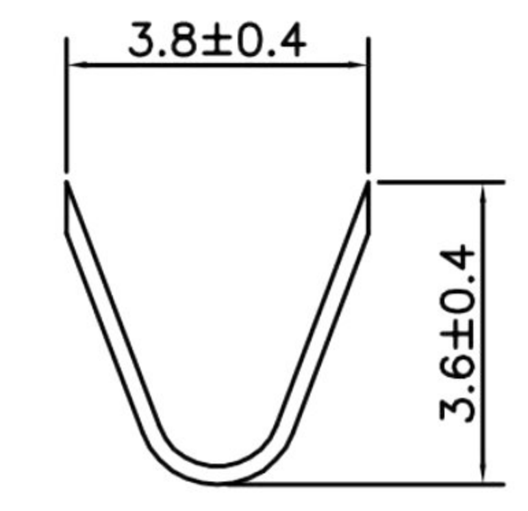
A-A Section
