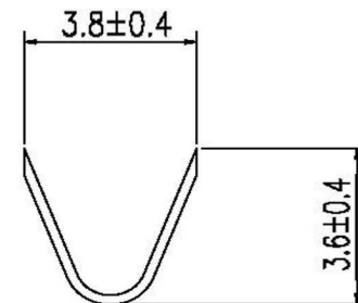
A-A Section
