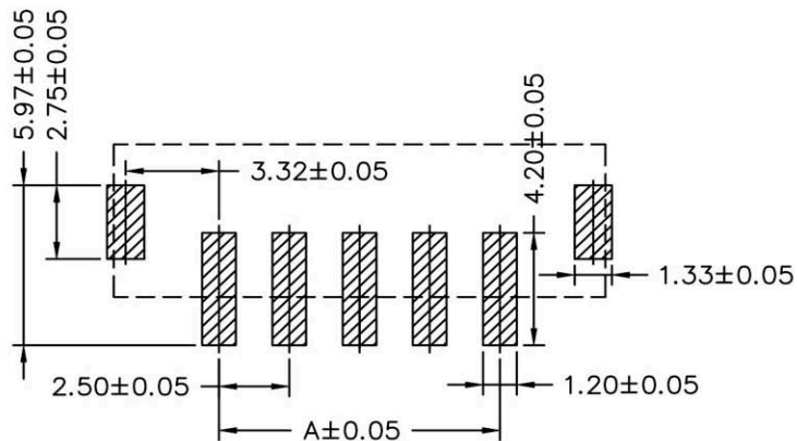
P.C.B LAYOUT
